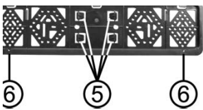
Figura 6: Montaggio targa
