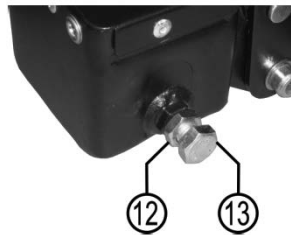
Bild 11: Einstellschraube
