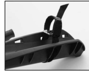
Bild 14: Montage Spanngurte
