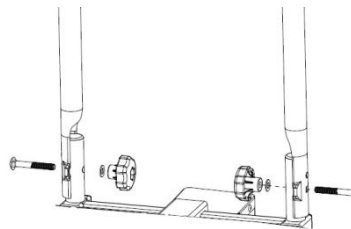
Bild 2: Montage U-Bügel
