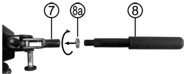
Bild 7: Montage Spannhebel
