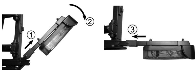
Bild 12: Verriegelung Leuchtenträger
