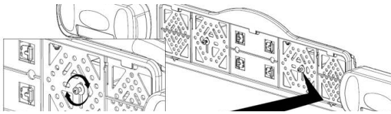
Bild 5: Montage Kennzeichenhalter
