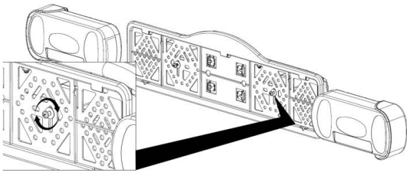
Figura 5: Montaggio portatarga
